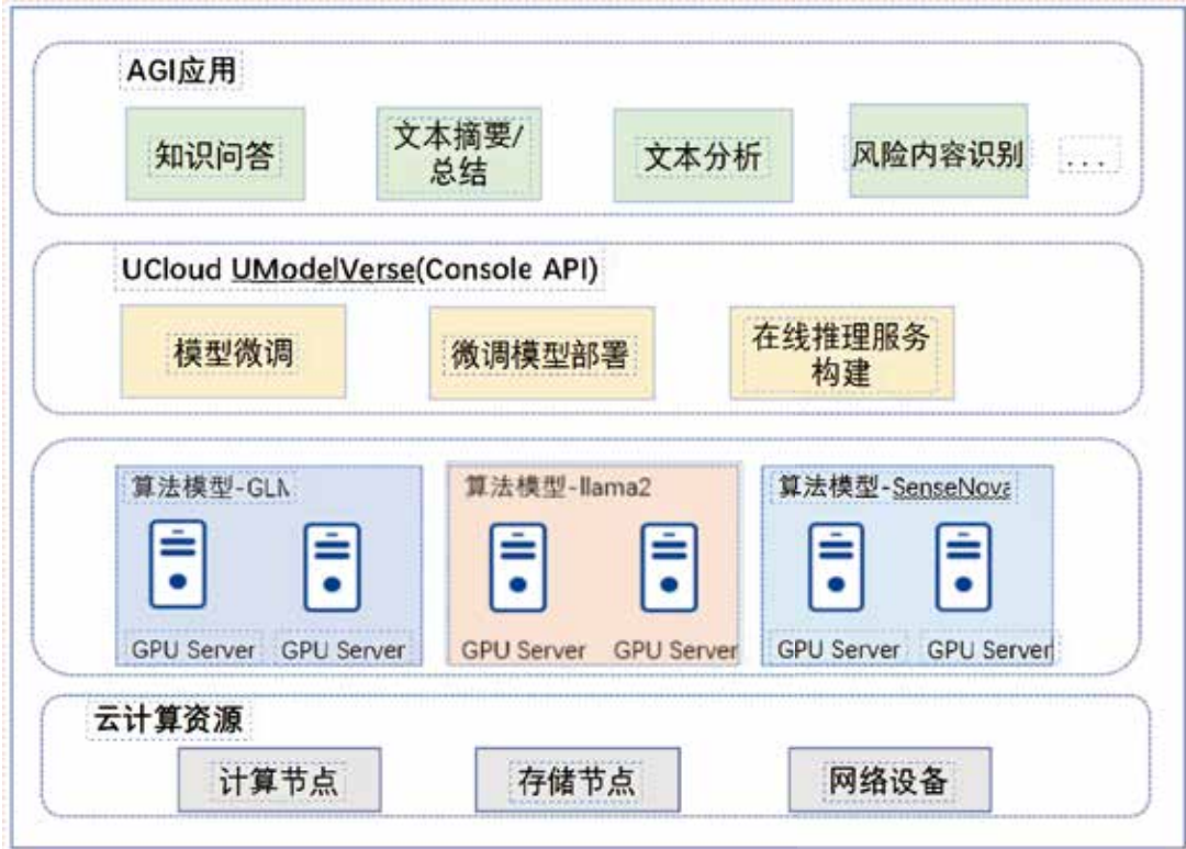
图3 UCloud-AGI 服务架构图
